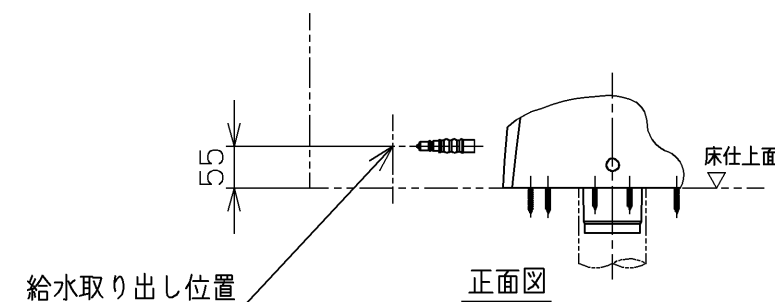
床給水仕様の場合
